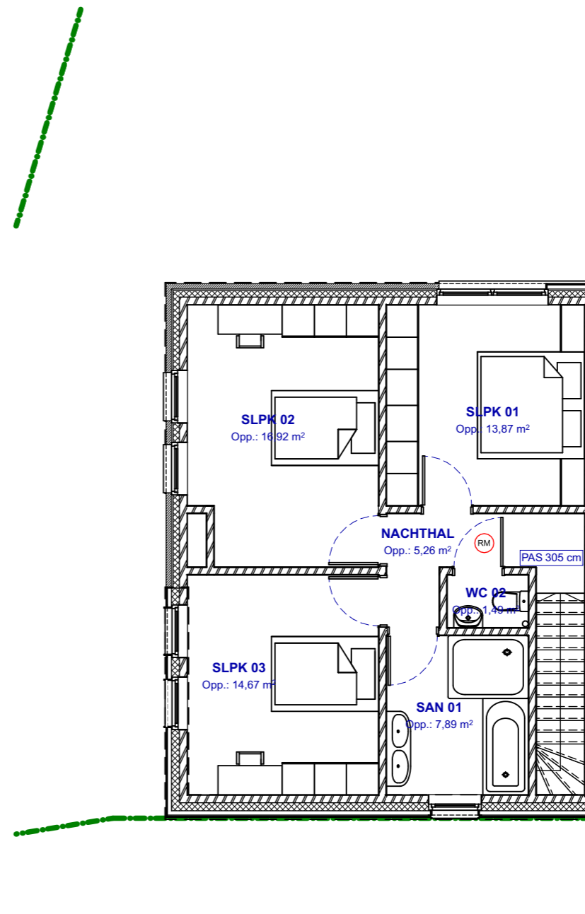
W08 NIVO +1 1:100
