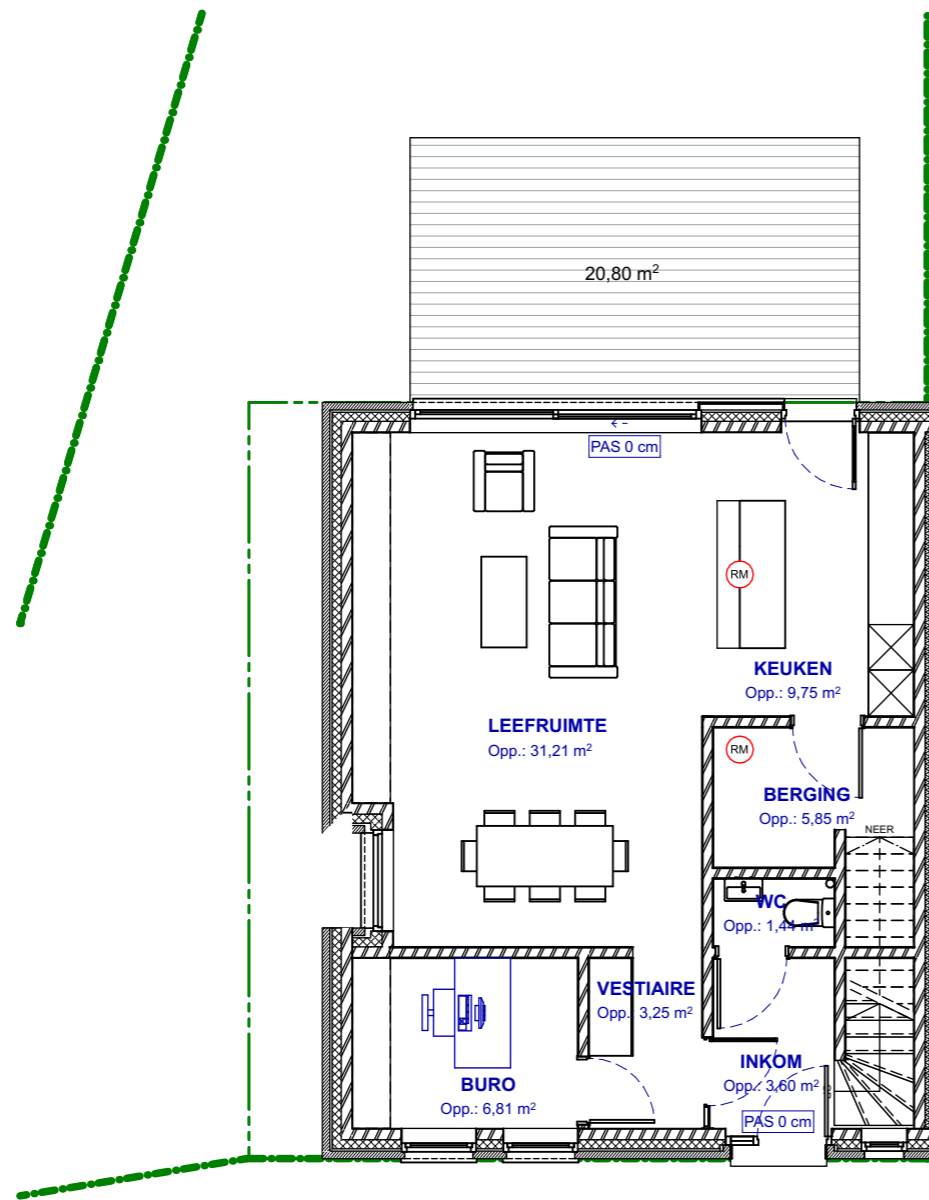
W08 NIVO +0 1:100
