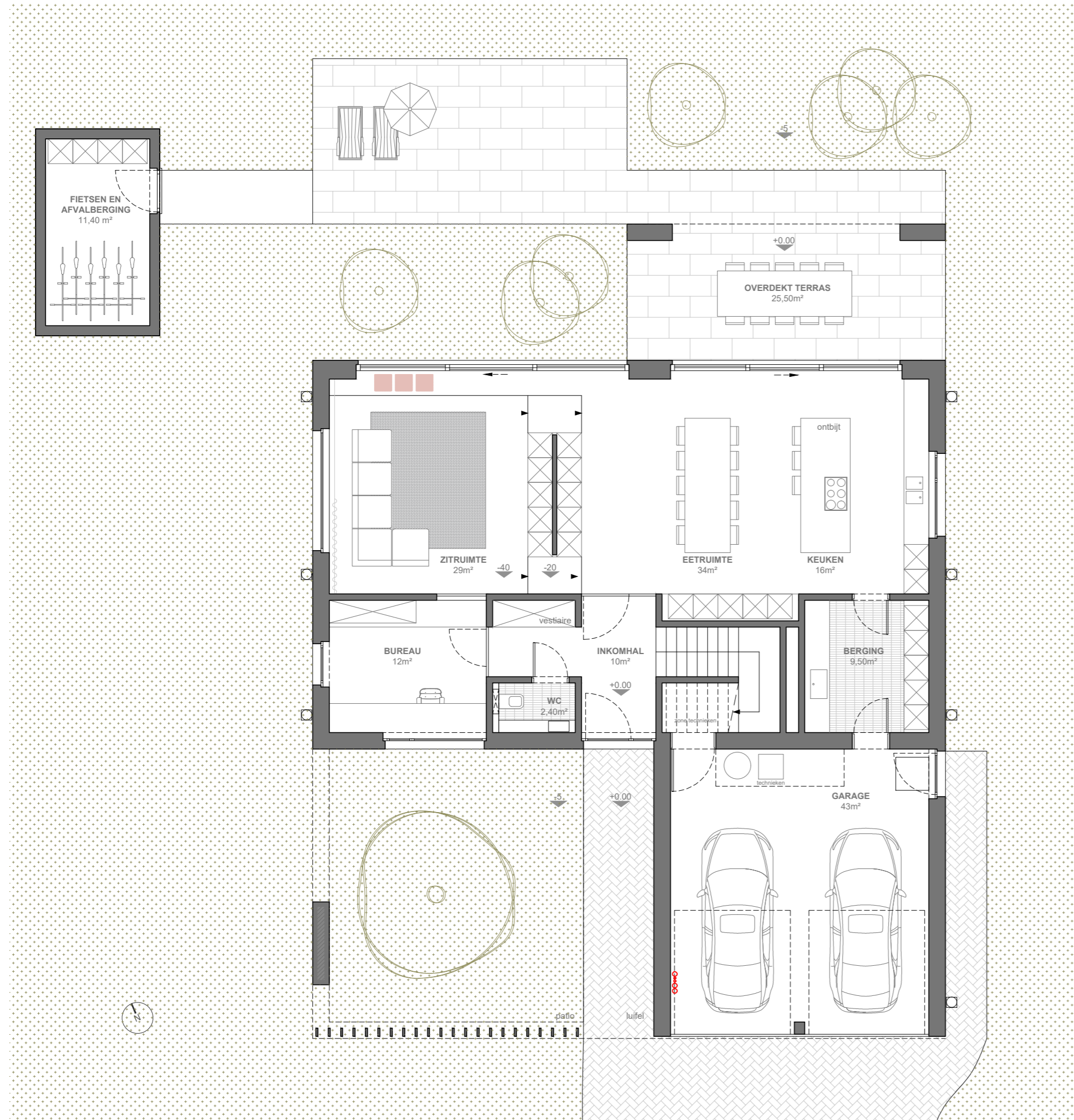
NIVEAU +00
